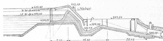
Abb. 1. Schnitt durch den Heber-Ueberlauf. — Masstab 1:1000.
