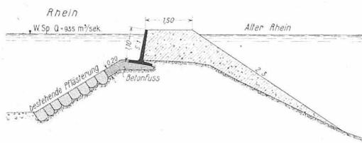
Abb. 11. Normalprofil der Uferverbauung mit Betonplatten. Masstab 1:150.
