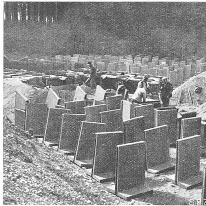
Abb. 9. Betonieren der Betonplatten System Schaub in der Kiesgrube Flaach.
