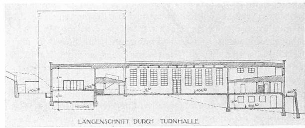
LÄNGENSCHNITT DURCH TURNHALLE
