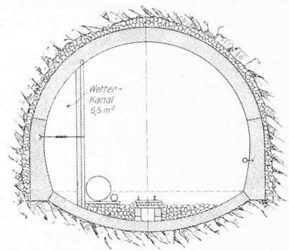
Abb. 6. Profil des zweispurigen Tunnels, links der Wetterkanal für den Bau. — 1:200.
