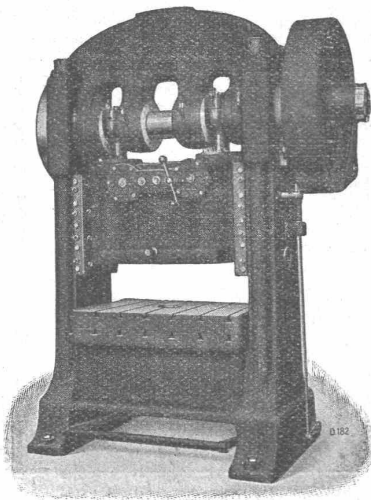
Doppelständer-Excenterpresse
