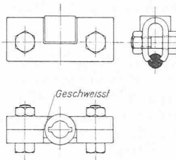
Abb. 19. Fahrdrabtklemme zum Spurhalterstab. 1 : 4.
