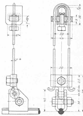
Abb. 16. Hängedrahtklemmen alter Bauart (Strecke Basel-Chiasso). Verschiedene Klemmen für Tragseil und Fahrdrabt. 1 : 4.
