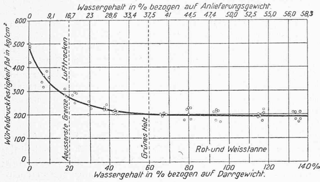
Abb. 2. Würfelfestigkeit. Abnahme der \beta_{\beta} mit zunehmendem Wassergehalt für Weiss- und Rottanne aus dem Kanton Zürich.
