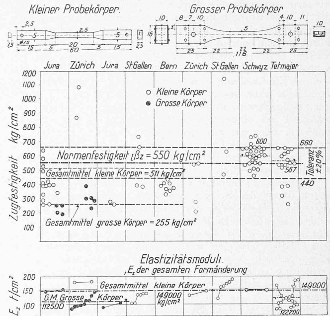
Abb. 1. Zugfestigkeiten und Elastizitätsmoduli von lufttrockener Tanne aus verschiedenen Gegenden der Schweiz.
