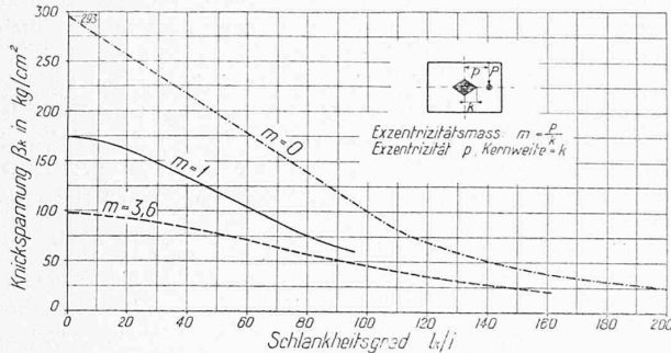
Abb. 4. Knicksfestigkeit. Einfluss des exzentrischen Kraftangriffs.
