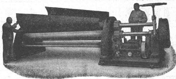
Vierwalzen-Blechrund- oder Biegemaschine
