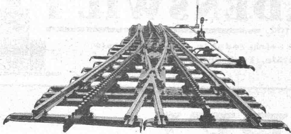
Aiguille pour voie à crémaillère
