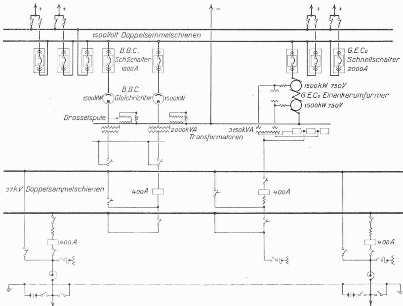
Abb. 4. Generelles, einpoliges Schaltungsdiagramm der Harvey-Unterstation.
