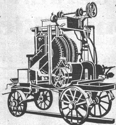
Fahrbarer Dampf- und Mörtemischer
