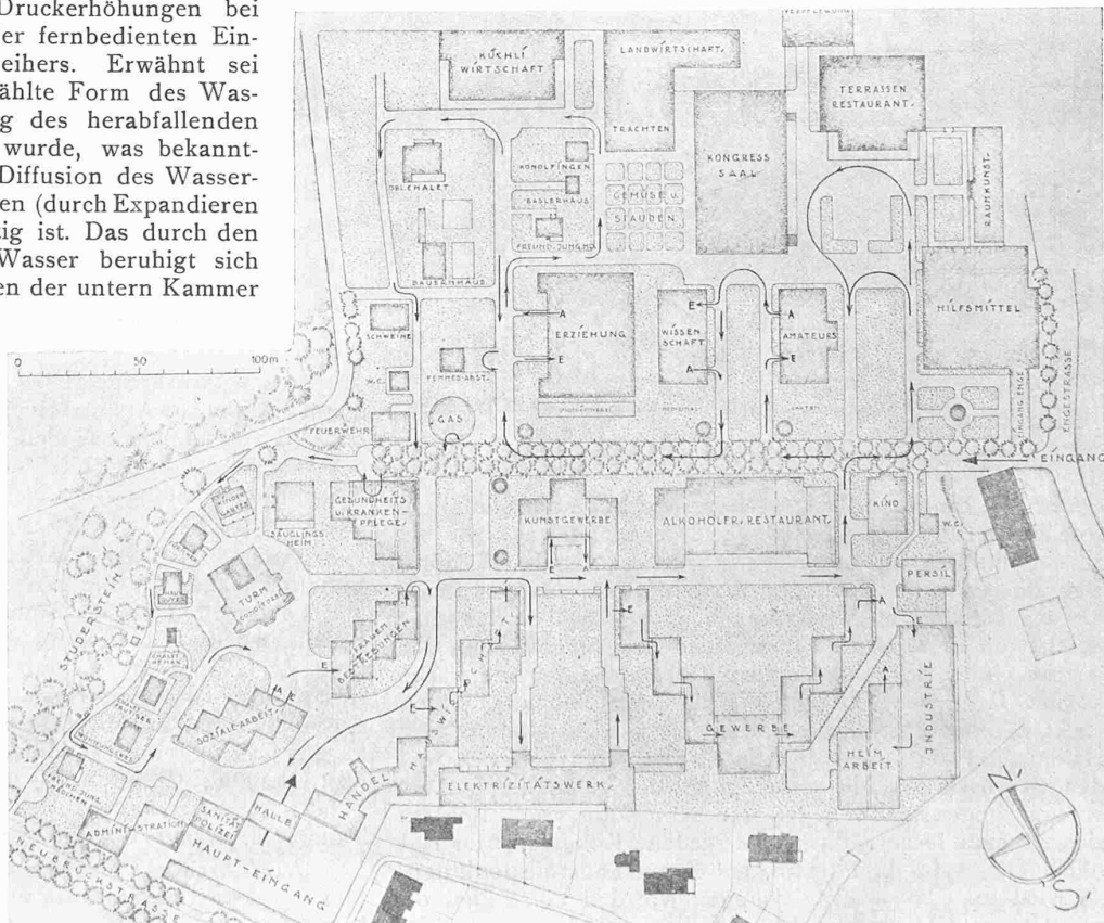
Abb. 1. Lageplan der „Saffa“, Schweizer. Ausstellung für Frauenarbeit. — 1 : 3000.
