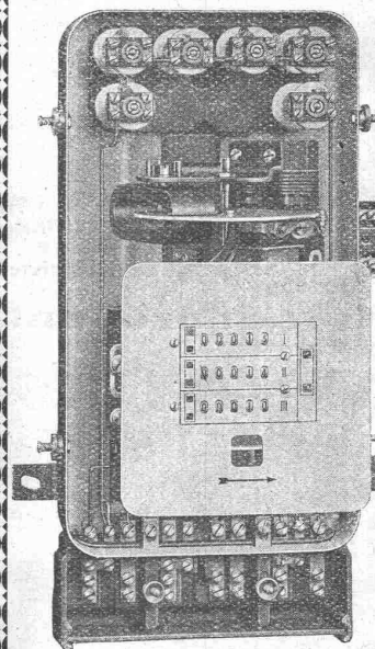
Dreifachtarif-Zähler
