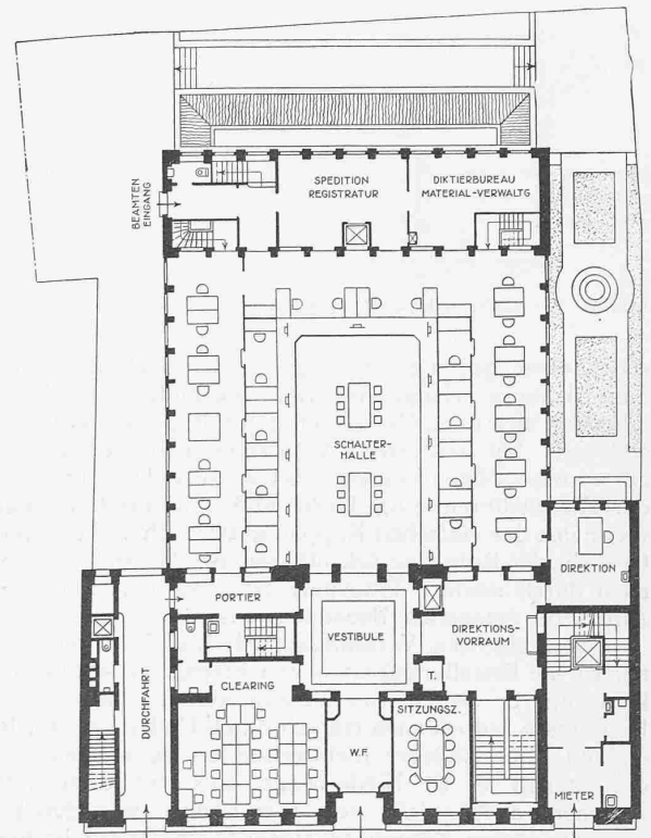
Abb. 2. Erdgeschoss-Grundriss. — Masstab 1 : 400.
