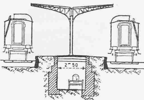
Abb. 7. Gepäck-tunnel mit Förderband unter den Anknft-Perrons der Fernzüge.
