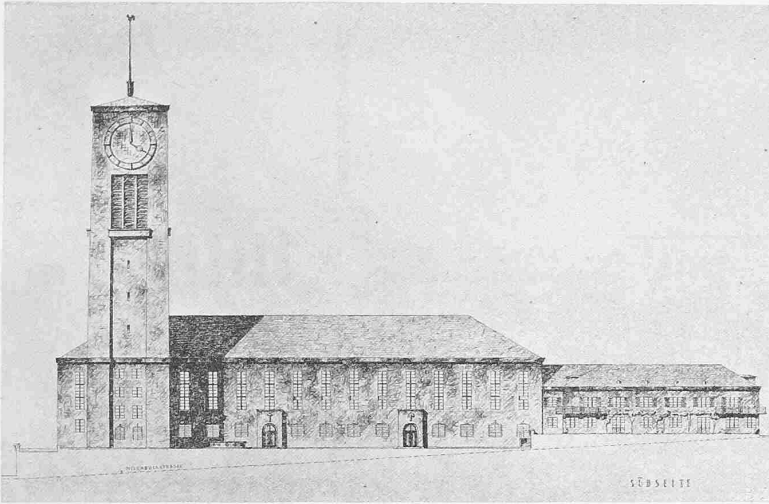
4. Rang (2300 Fr.), Entwurf Nr. 8. — Architekt Martin Risch, Zürich. — Süd- und Westansicht, 1 : 1000.
