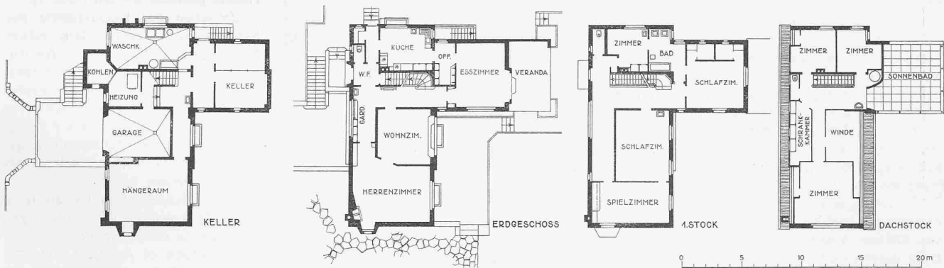
Abb. 4. Grundrisse, Masstab 1 : 400.
