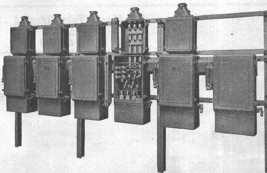
Gusseiserngekapselte Niederspannungs-Verteilanlage.
