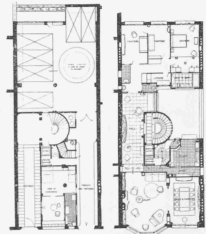
Abb. 1 und 2. Grundrisse 1 : 400.
