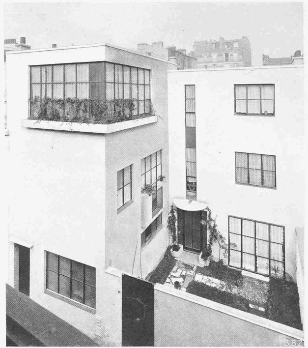
Abb. 10. Ansicht des Hauses J. Lurçat von der Strassen-(Garten-)Seite.
