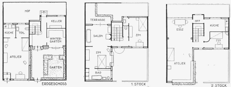
Abb. 6 bis 8. Grundrisse des Hauses von Kunstmaler Jean Lurçat.
