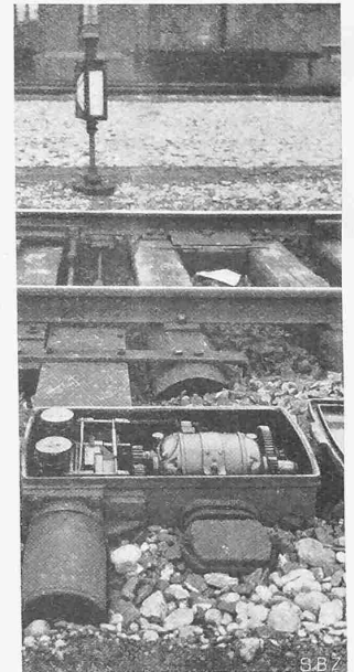
Abb. 16. Elektr. Weichenantrieb. Konstruktionen der „Signum A.-G.“ Wallisellen bei Zürich.
