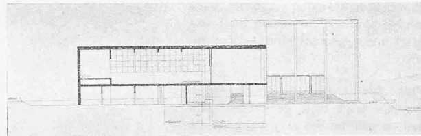
Längsschnitt durch den Gemeindesaal und Grundriss vom Obergeschoss, 1 : 800. Oben Süd- und West-Fronten.
