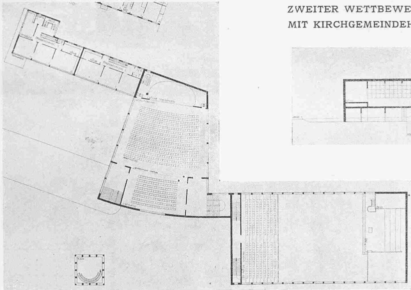
Längsschnitt durch den Gemeindesaal und Grundriss vom Obergeschoss, 1 : 800. Oben Süd- und West-Fronten.
