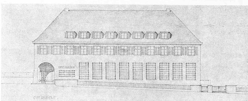
Ostfassade 1 : 400.
