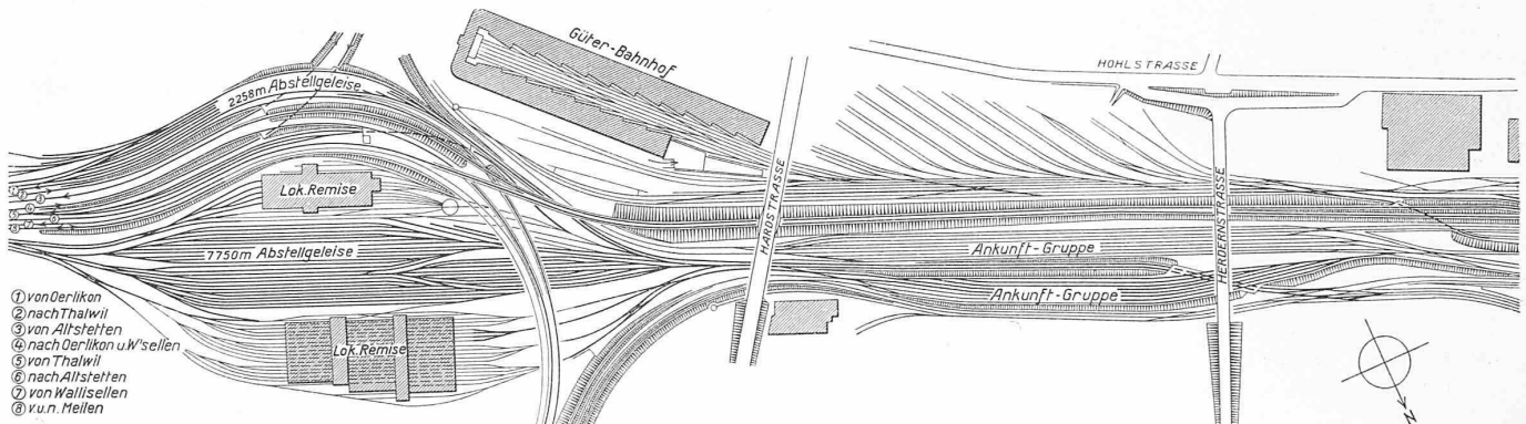
Abb. 9. IV. Etappe (östl. Teilstück): Personen-Abstellgeleise, Verlegung der Personen-Hauptgeleise Richtung Altstetten vom Nordrand gegen Süden mit zahlreichen Ueberwerfungen zur kreuzungsfreien Einführung aller Linien. — Masstab 1:10000.
