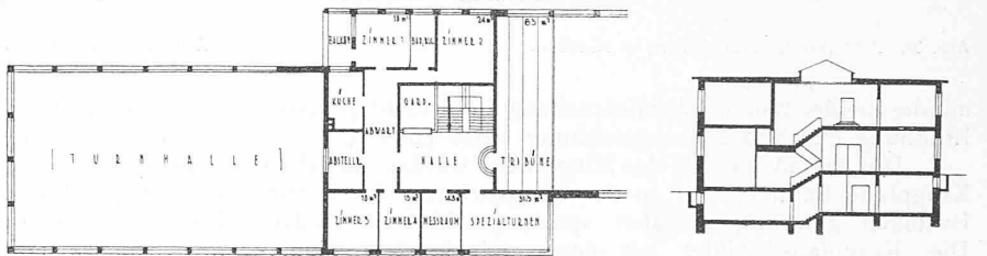
1. Rang (2200 Fr.), Entwurf Nr. 10. — Verfasser Scherrer & Meyer, Architekten, Schaffhausen. Ansicht der Doppelturnhalle aus Südwest. — Grundrisse und Querschnitt 1 : 600.
