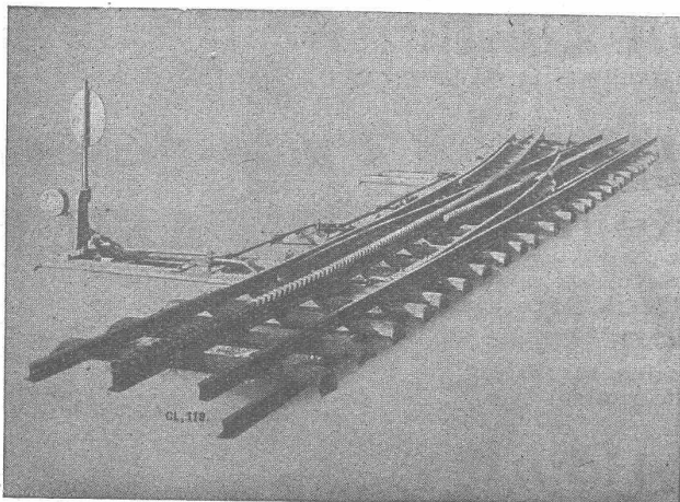
Zahnstangenweiche Jungfraubahn.
