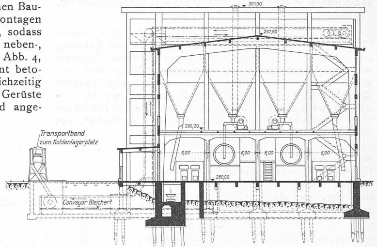
Abb. 6. Querschnitt Süd-Nord durch die Kohlentrocknerei. — Masstab 1 : 400.
