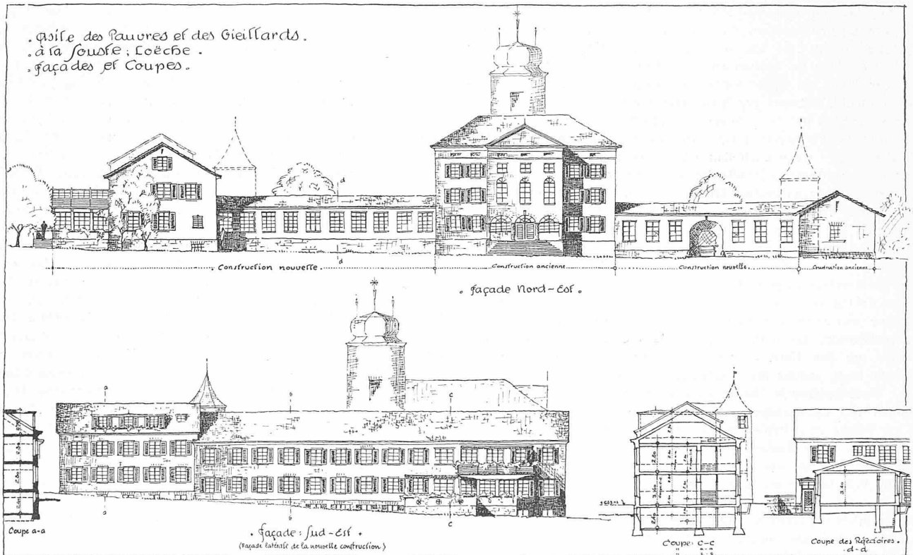
I. Preis (2000 Fr.), Entwurf Nr. 5. Verfasser Arch. Jos. Stöcklin, Neualschwyl (Basel). — Fassaden und Schnitte 1 : 500. (Plan-Clichés des „Bulletin Technique“.)
