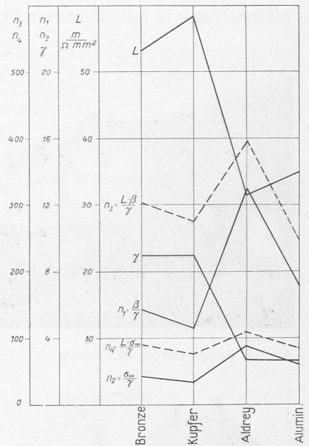
Abb. 1. Bruchfestigkeit β, Streckgrenze σ, Elastizitätsgrenzen für Dehnungen 0,05 u. 0,01, Dehnung λ. Abb. 2. Elektrische Leitfähigkeit L, spezifisches Gewicht λ, Verhältniszahlen n 1 , n 2 , n 3 und n 4 .
