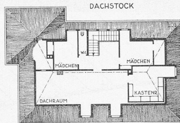
Abb. 6 bis 9. Grundriss 1 : 400 zum HAUS WEGMANN-RUCH IN ZÜRICH.
