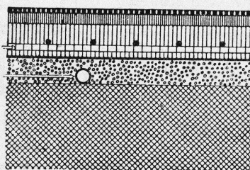
Patentierte „Isolaphon“-Unterlagsboden
