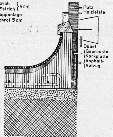
Patentierter „Isolaphon“-Unterlagsboden
