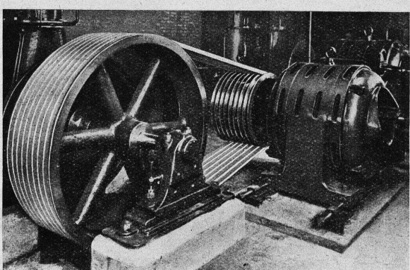
Antrieb eines Kompressors, 130/150 PS.
