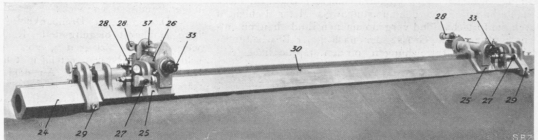
Abb. 5. Horizontal-Komparator mit zwei Mess-Schlitten für Längenmessungen; Beobachterseite.
