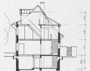
Abb. 9 bis 11. Grundrisse und Schnitt, 1 : 400.
