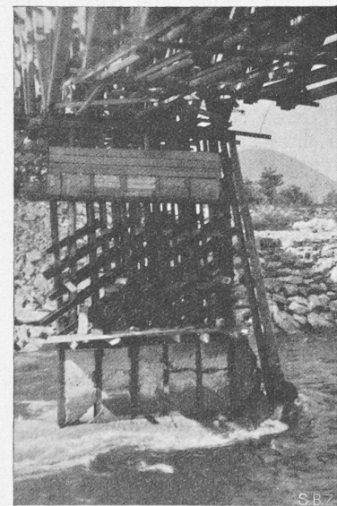
Abb. 1. Die planwidrige Pendelstütze, kurz vor dem Einsturz, den statt der vorgesehenen Ausbetonierung nachträglich aufgeklebte (!) Diagonalen noch hätten aufhalten sollen.
