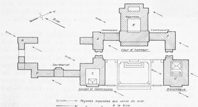
Abb. 12. Gruppen-Unterteilung der Heizung nach Projekt der Bauleitung.
