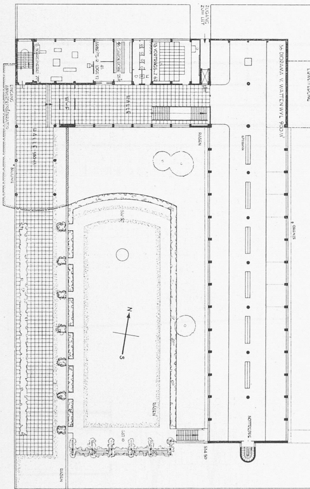
Erdgeschoss, darüber Längsschnitt durch die Eingangshalle. — 1 : 600.
