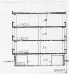
Sammlungsflügel. Schnitt. Masstab 1 : 600.
