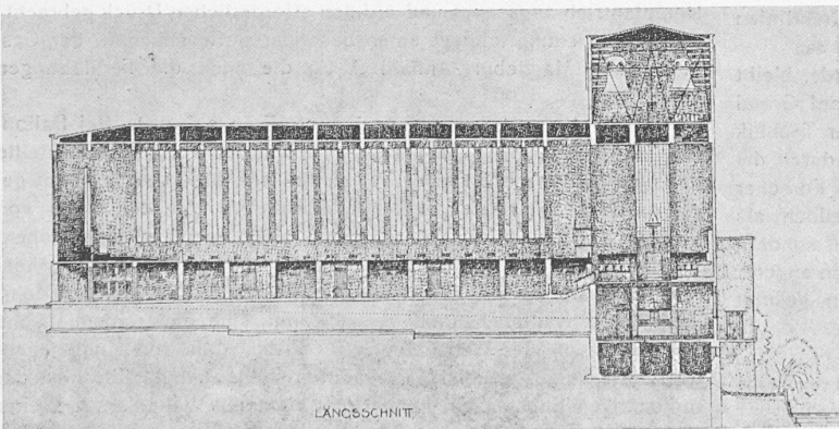
LÄNGSSCHNITT
