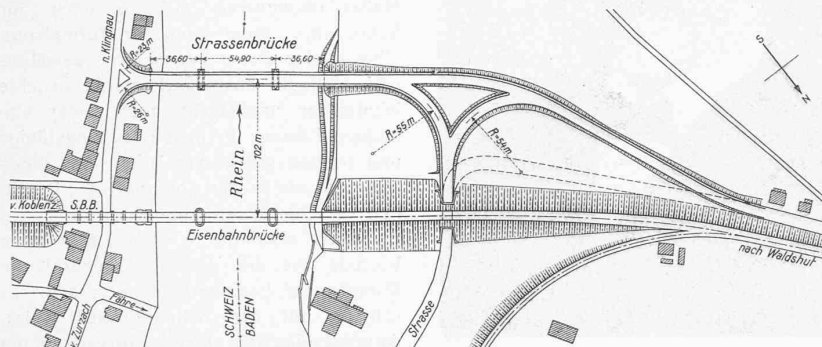
Abb. 1. Lageplan der Rheinbrücken Koblenz-Waldshut. — Masstab 1 : 5000.
