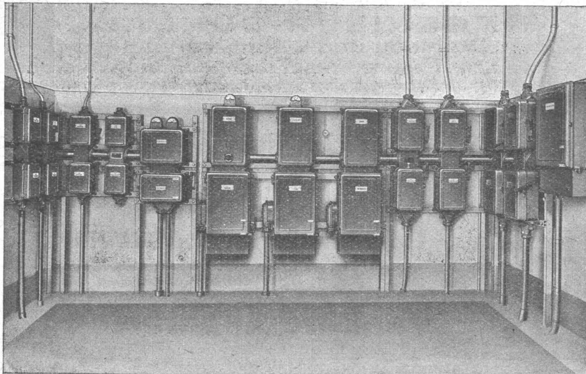
Gussgekapselte Niederspannungs-Verteilanlage
