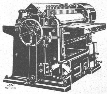
Hochleistungs-Dickenhobelmaschine Typ DH
