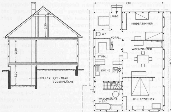
Abb. 1. Schnitt und Grundriss des Kleinhauses. — Masstab 1 : 200.
