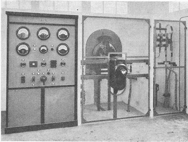
Abb. 12. Unterstation Niederteufen. Zellen für die ankommenden Linien und die Apparatur auf der Primärseite des Gleichrichter-Transformators.
