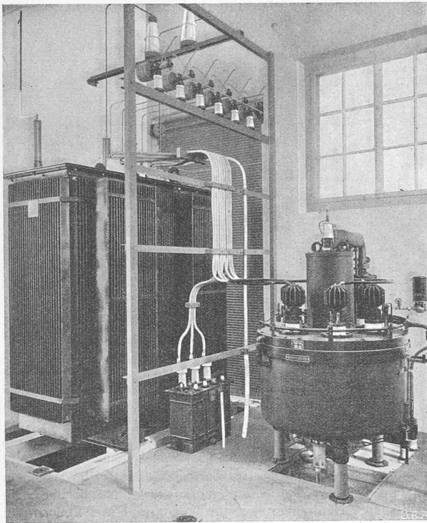
Abb. 14. Unterstation Gais. Gleichrichter mit Haupttransformator und Hilstransformator.
