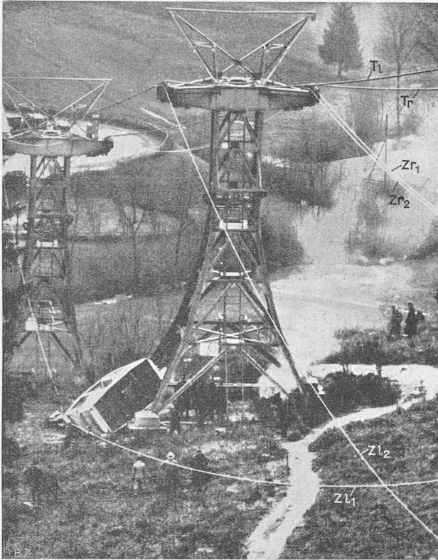
Die Absturzstelle am Mast Nr. 2 der Schauinsland-Bahn bei Freiburg i. Br., einer neuartigen Personen-Seilschwebebahn mit Umlaufbetrieb. T 1 u. Tr Tragseil links bzw. rechts, Z r Zugseilpaar links, Z r Zugseilpaar rechts. Photo A. Müller, Freiburg i. Br.
