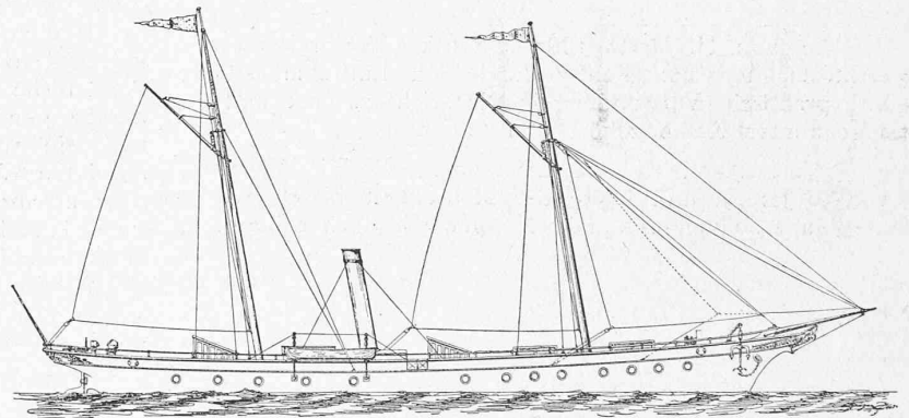
Abb. 69. Dampf-Segeljacht auf dem Genfersee, gebaut 1883 von Escher Wyss & Cie., Zürich [9. Aug. 1884]. Länge ü. A. 38,5 m, Breite 5,0 m, Déplacement 100 t; 250 PSi, n 135, v 24 km/h. — Das Schiff fährt heute als „Cadenabbia“ (mit Dieselantrieb) auf dem Comersee, als besonders seetüchtig beliebt.
