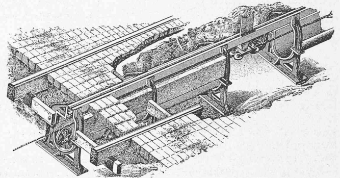
Abb. 67 und 68. A. S. Hallidies Strassenbahn mit umlaufendem Seil, erstmals in Betrieb gesetzt 1873 in San Francisco [„S. B. Z.“ 20. Januar 1883].
