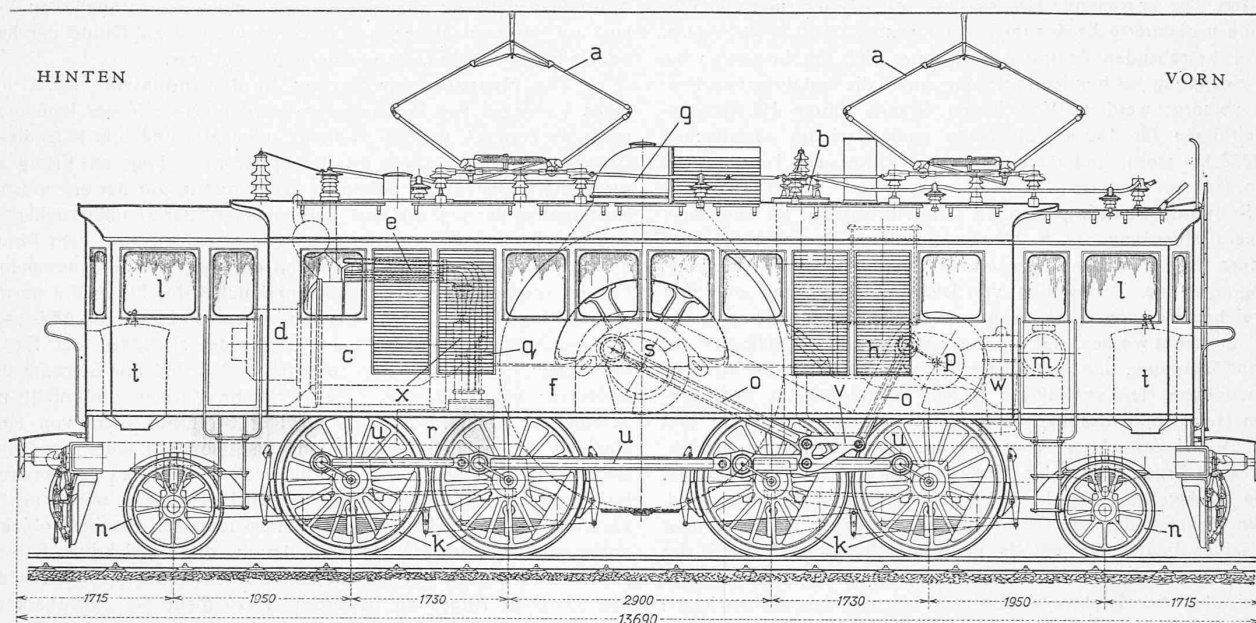
Einphasen-Drehstrom-Umformerlokomotive nach System Kandó für die ungarischen Staatsbahnen. — Masstab 1 : 75. (Vergl. unter Literatur auf S. 109 dieser Nr.)
