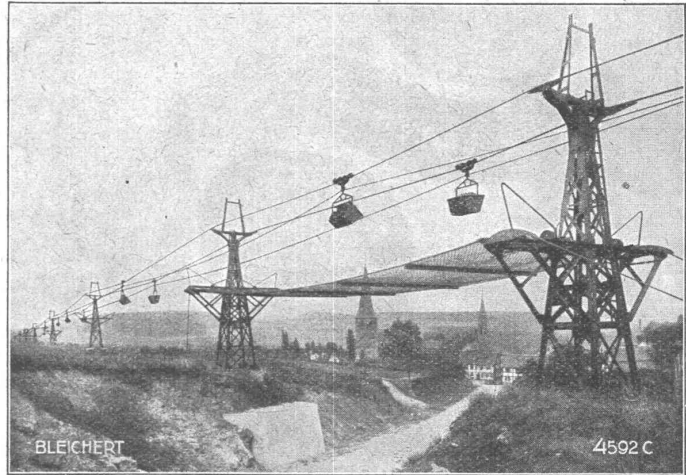
Drahtseilbahn von 2000 m Länge, 150 t/h Leistung der Rheinisch-Westfälischen Kalkwerke Dornap in Gruiton (Rheinland)
