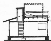
Abbildung 9. Schnitt.
