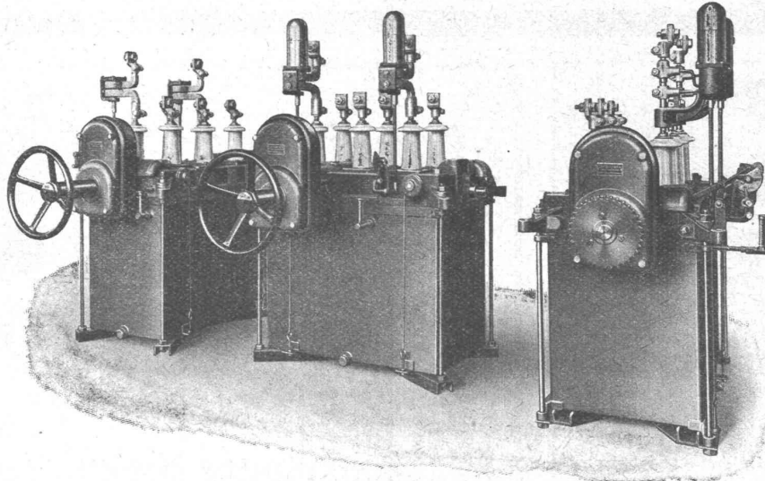
Dreipolige automatische Oelschalter Type 25 000 Volt 200 und 600 Ampère.
