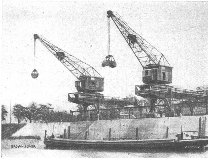
Neptun A.-G., Basel. Halbportalkrane von 5 t Tragkraft für Stückgut und Greiferbetrieb im Rheinhafen.
